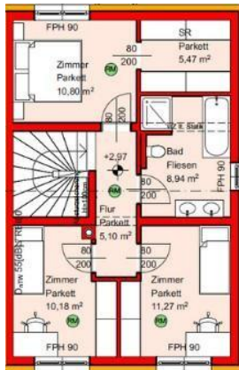
Grundriss OG Top 3
